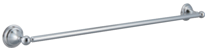
122 タオルバー GSN-2112201A クローム 設計価格 ¥11,600 W660 × D70 × H60mm 耐荷重：4kg
